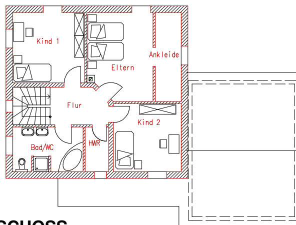
OBERGESCHOSS
